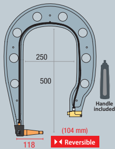
G4 8 bar/550 daN 022799
