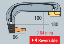
G1 8 bar/550 daN 022768
