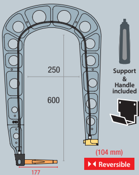
G10 8 bar/400 daN 067165
